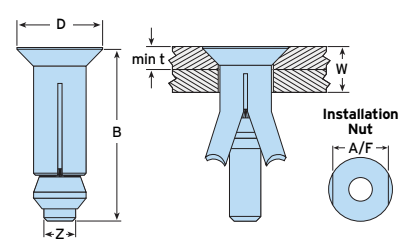
c) Flush Fit
